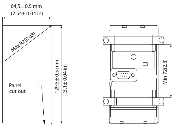
Рисунок 11.29 Размеры
