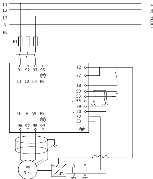
Рисунок 10.7 Пример подключения регулятора скорости
