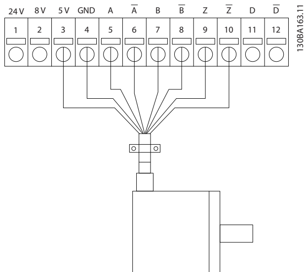
Рисунок 11.3 Инкрементальный энкодер
