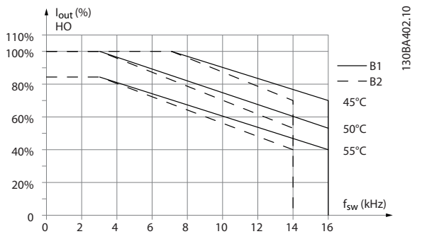
Рисунок 6.6 Снижение номинального тока I_{\text{вых}} при различных значениях T_{\text{ОКР. СР. МАКС}} для корпусов типа B1 и B2 и модели коммутации 60° AVM в режиме высокой перегрузки (крутящий момент 160 %)
