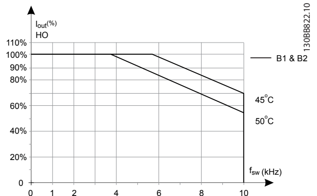
Рисунок 6.15 Снижение номинального выходного тока при частотах коммутации и окружающей температуре для преобразователей частоты на 600 В с типом корпуса B и моделью коммутации 60° AVM в режиме высокой перегрузки
