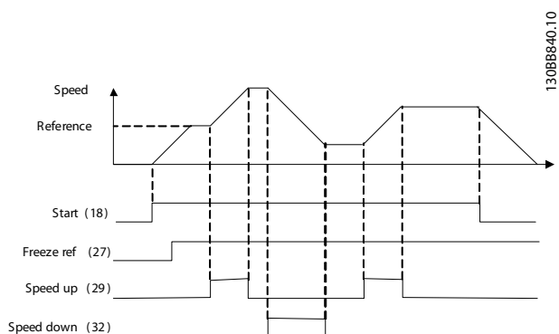
Рисунок 10.3 Увеличение/снижение скорости
