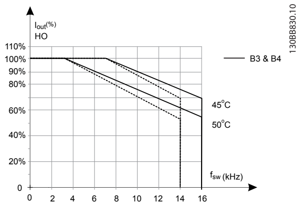
Рисунок 6.8 Снижение номинального тока I_{\text{вых}} при различных значениях T_{\text{ОКР. СР. МАКС}} для корпусов типа B3 и B4 и модели коммутации 60° AVM в режиме высокой перегрузки (крутящий момент 160 %)
