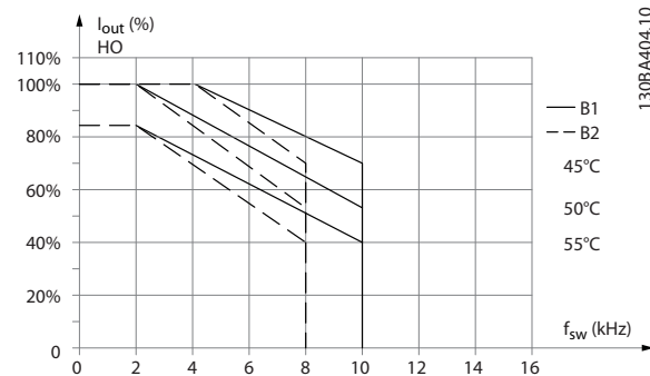
Рисунок 6.10 Снижение номинального тока I_{\text{вых}} при различных значениях T_{\text{ОКР. СР. МАКС}} для корпусов типа B1 и B2 и модели коммутации SFAVM в режиме высокой перегрузки (крутящий момент 160 %)
