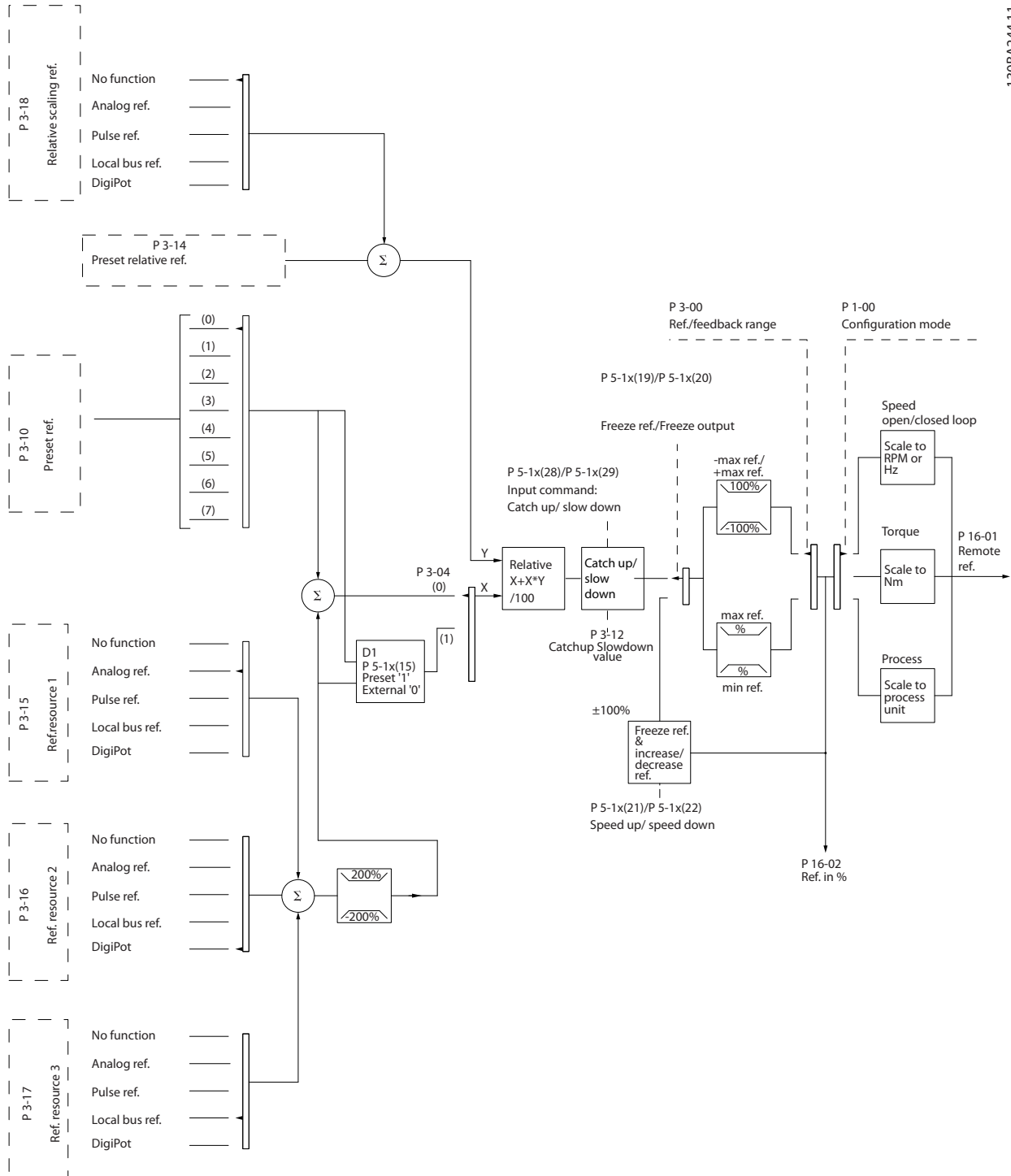
Рисунок 3.13 Дистанционное задание
