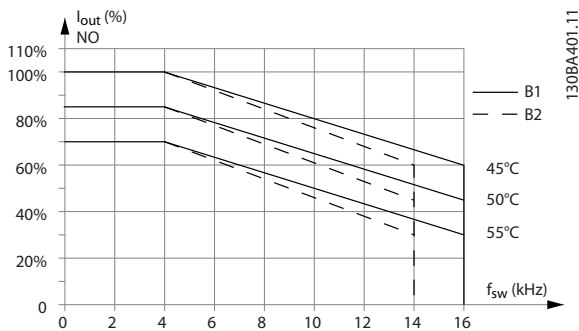
Рисунок 6.7 Снижение номинального тока I_{\text{вых}} при различных значениях T_{\text{ОКР. СР. МАКС}} для корпусов типа B1 и B2 и модели коммутации 60° AVM в режиме нормальной перегрузки (крутящий момент 110 %)
