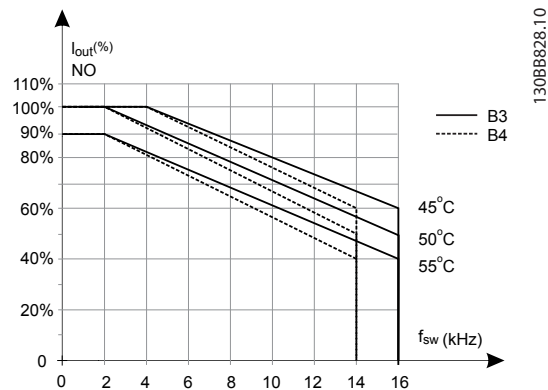
Рисунок 6.9 Снижение номинального тока I_{\text{вых}} при различных значениях T_{\text{ОКР. СР. МАКС}} для корпусов типа B3 и B4 и модели коммутации 60° AVM в режиме нормальной перегрузки (крутящий момент 110 %)
