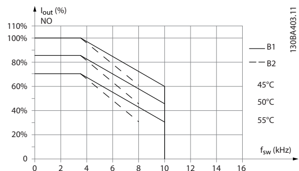
Рисунок 6.11 Снижение номинального тока I_{\text{вых}} при различных значениях T_{\text{ОКР. СР. МАКС}} для корпусов типа B1 и B2 и модели коммутации SFAVM в режиме нормальной перегрузки (крутящий момент 110 %)
