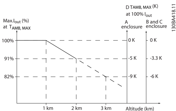
Рисунок 5.1 Снижение номинального выходного тока в зависимости от высоты над уровнем моря при температуре окружающей среды T_{\text{окр. ср.}} , МАКС. для типоразмеров А, В и С. При высоте более 2000 м свяжитесь с Danfoss по вопросам защитного сверхнизкого напряжения.
