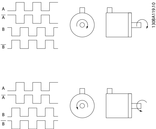
Рисунок 11.5 Направление вращения
