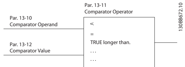
Рисунок 4.6 Компараторы
