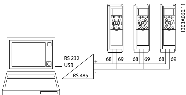
Рисунок 12.2 Параллельные соединения
